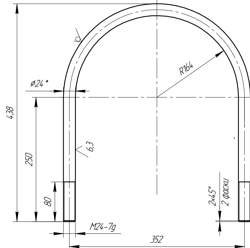
Дет. поз. 5
