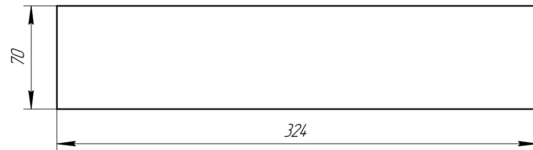
Дет. поз. 4 (1:2,5)
