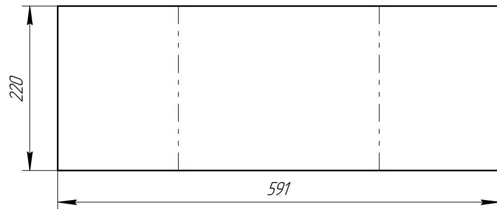
Дет. поз. 2 (1:2)
